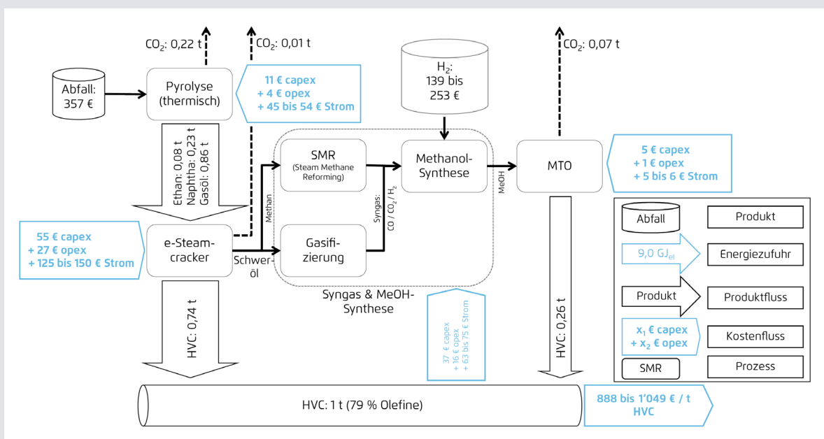
Abbildung 2: Vereinfachtes Kostenflussdiagramm für 2050 und die integrierte Route von Pyrolyse, elektrischem Steamcracking und MTO
