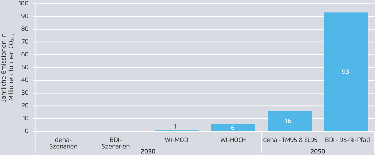
Vergleich des jährlichen Umfangs der CO 2 -Abtrennung an Industrieprozessen und Speicherung (CCS) in den Szenarien MOD und HOCH im Vergleich mit anderen Szenarien aus der Literatur
